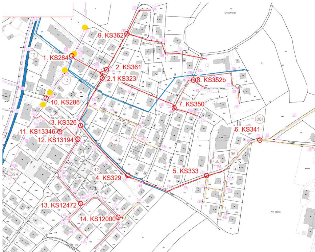
Auszug Skizze Fremdwassermessungen, Porta AG, 26.06.2024 / blp
